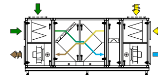
Yhd. 9 Vastavirtalämmönsiirrin ja kiertoilmaosa
