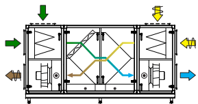
Yhd. 7 Vastavirtalämmönsiirrin
