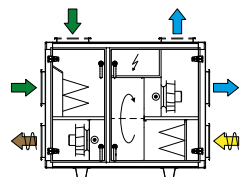
Tuloilma ylhäältä
