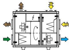
Tuloilma alhaalta
