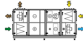
Yhd. 12 Patteritalteenotto-osa ja jäähdytyslaite
