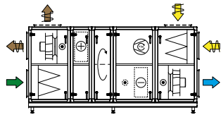
Yhd. 3 Jäähdytyslaite jäähdytysenergian talteenotolla
