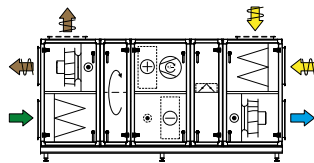
Yhd. 5 Roottori, jäähdytyslaite ja sekoitusosa
